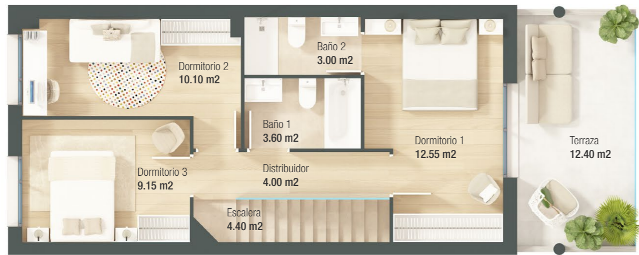
PLANTA PRIMERA
